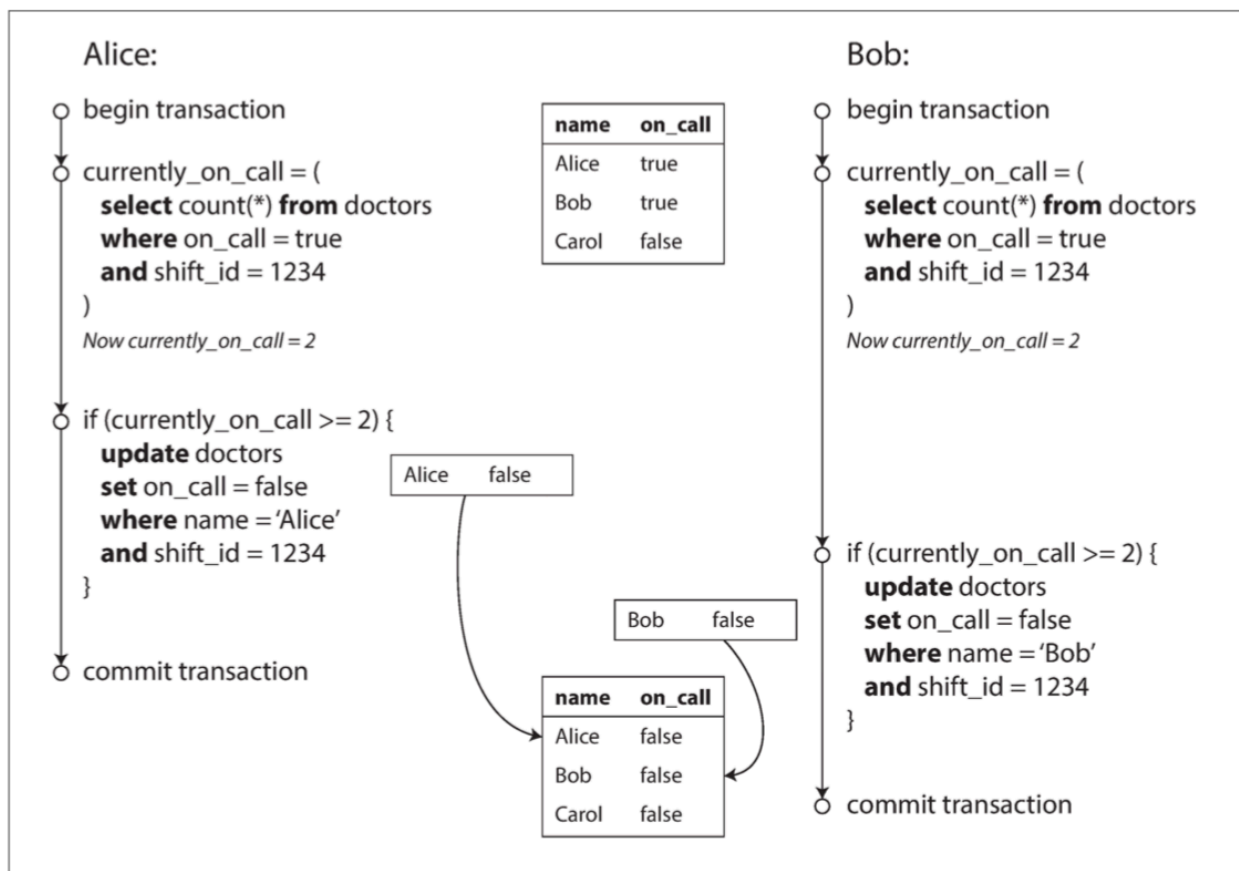
图 13: Write Skew
