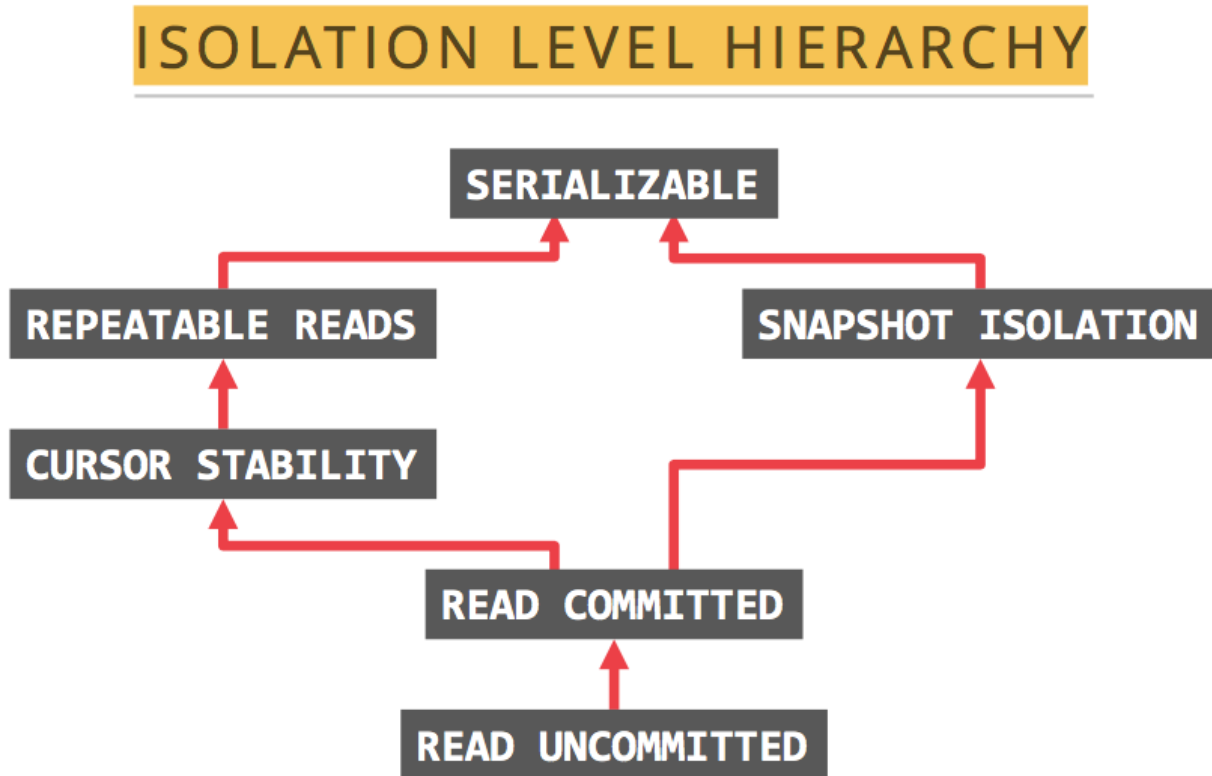
图 12: 隔离级别
