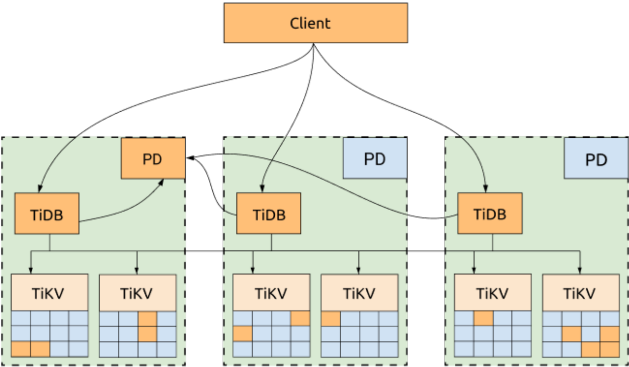
图 1: 三 AZ 部署
