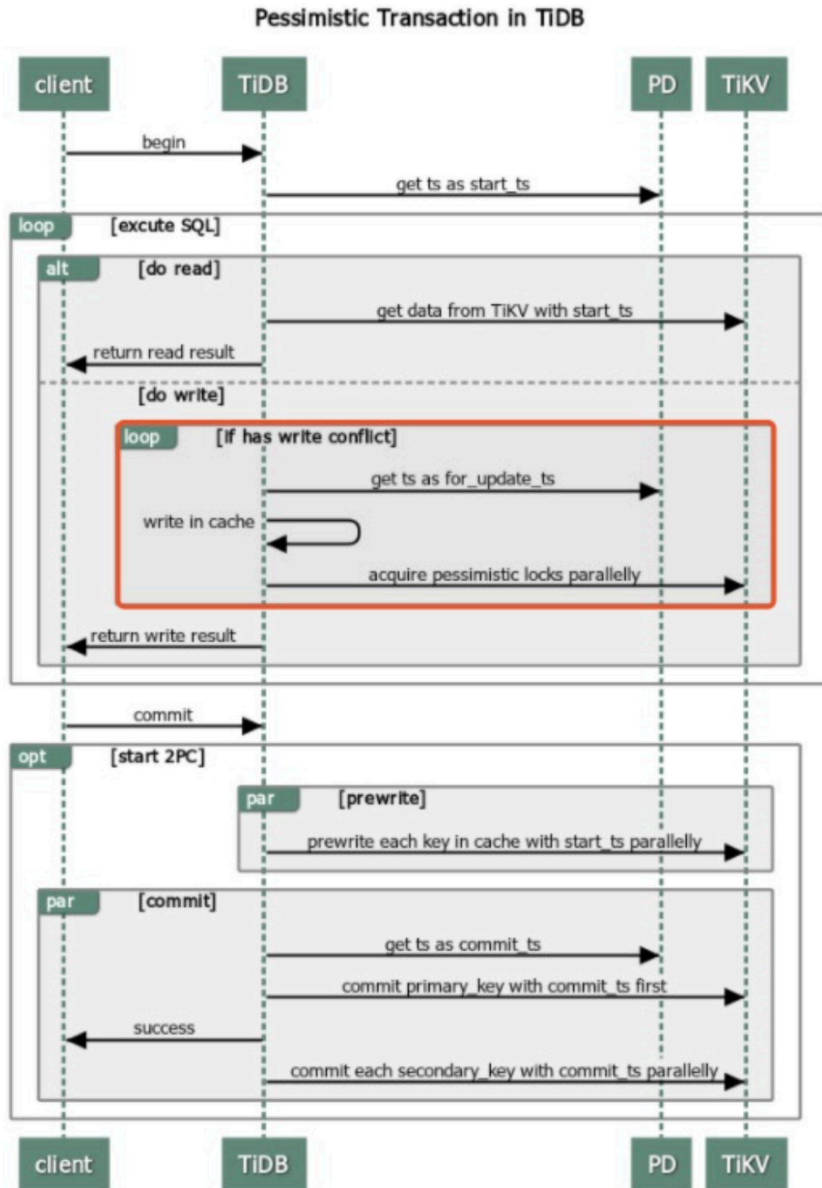
图 215: 平凯数据库中的悲观事务
