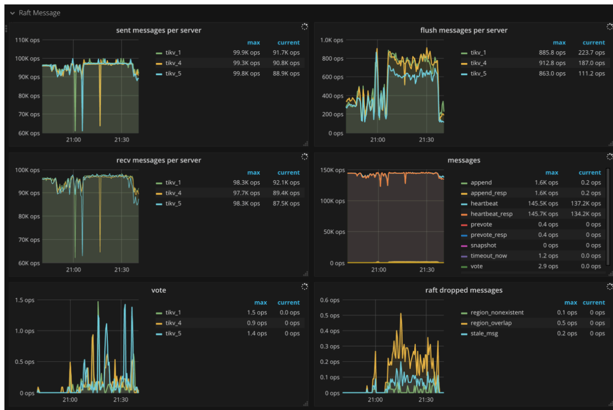
图 69: TiKV Dashboard - Raft message metrics
