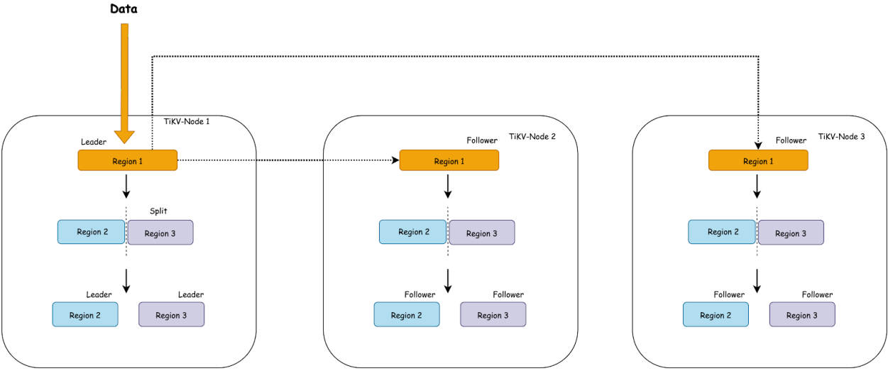
图 16: TiKV Region 分裂流程
