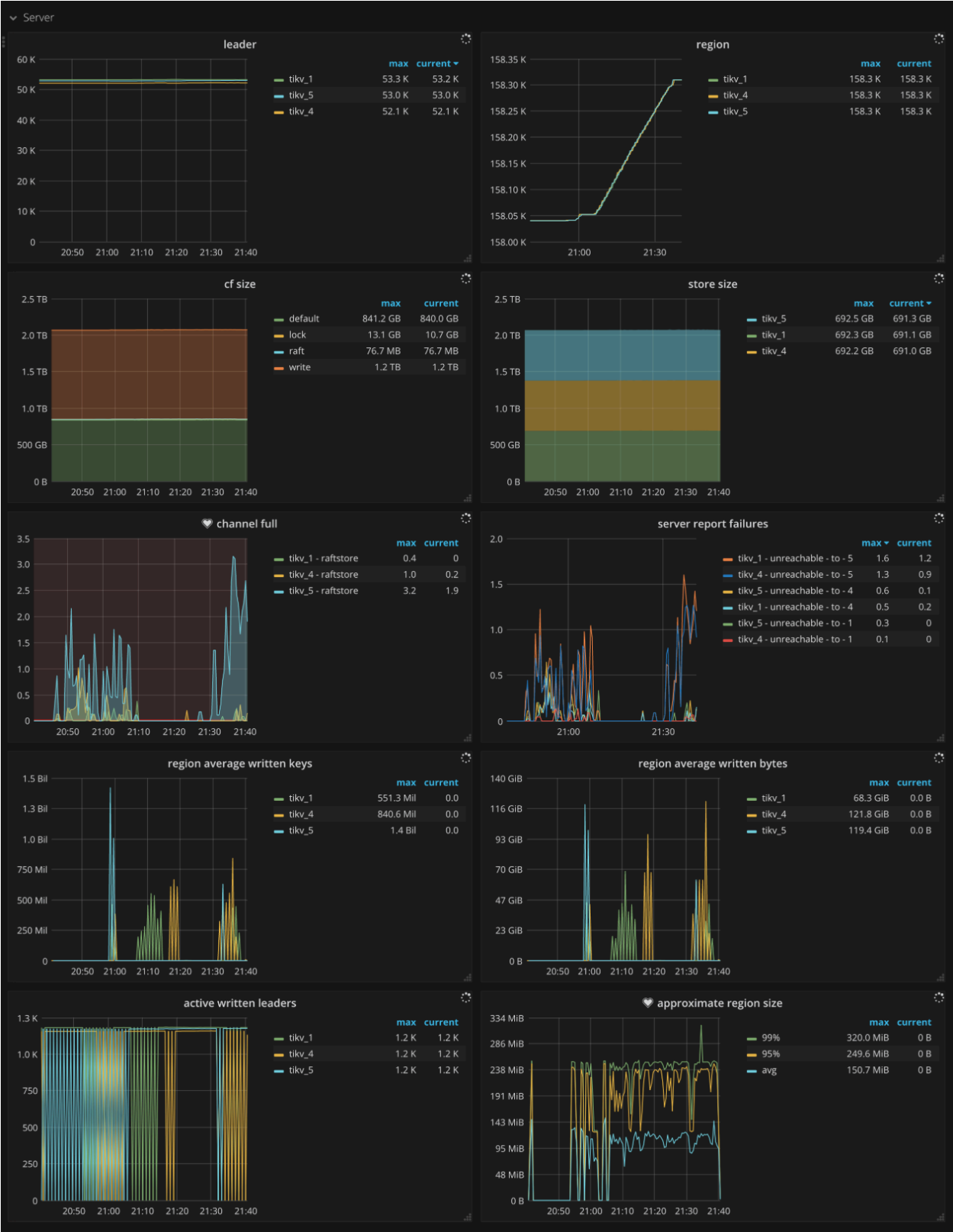
图 66: TiKV Dashboard - Server metrics
