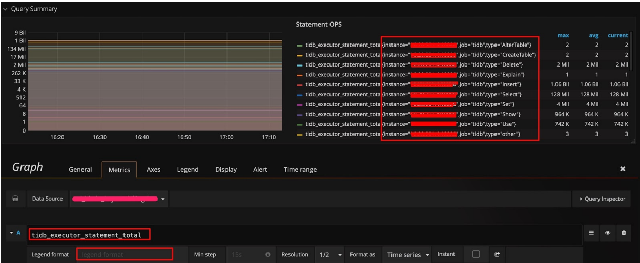
图 25: 编辑表达式并查看所有维度
