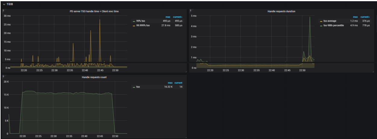
图 61: PD Dashboard - TiDB node metrics
