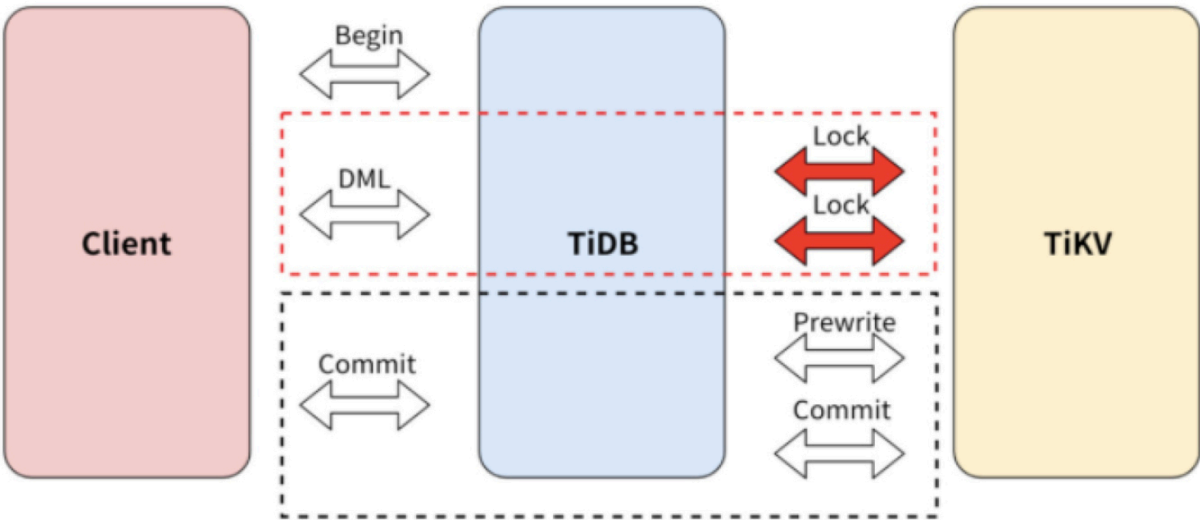
图 214: 平凯数据库悲观事务的提交流程
