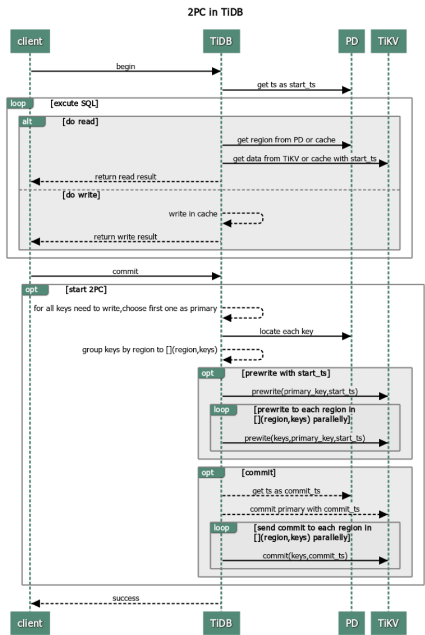
图 212: 平凯数据库中的两阶段提交
