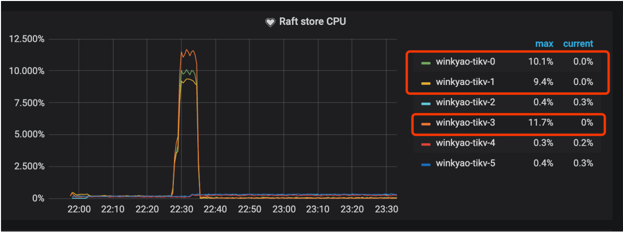
图 14: QPS3
