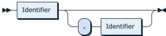
图 203: TableName
