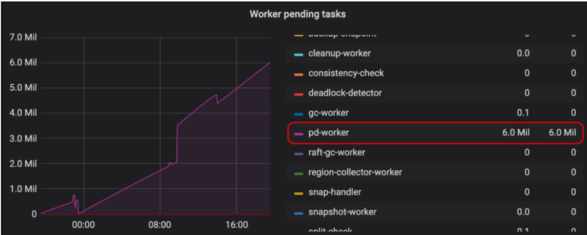
图 41: 图 4 查看 pd-worker
