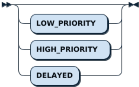
图 205: PriorityOpt
