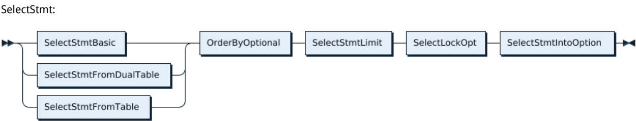
图 83: SelectStmt
