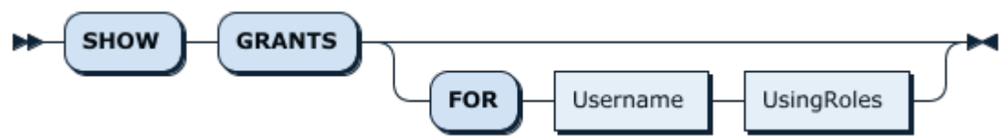
图 143: ShowGrantsStmt
