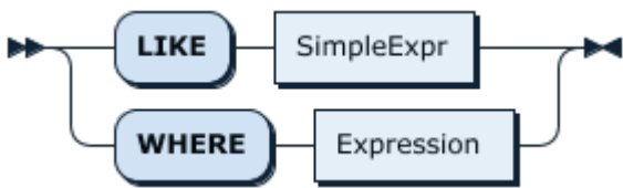
图 116: ShowLikeOrWhereOpt
