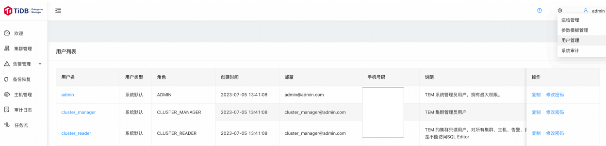
图 253: 用户管理
