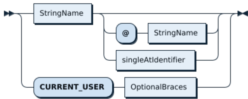
图 144: Username
