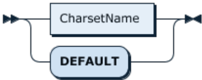
图 106: CharsetNameOrDefault
