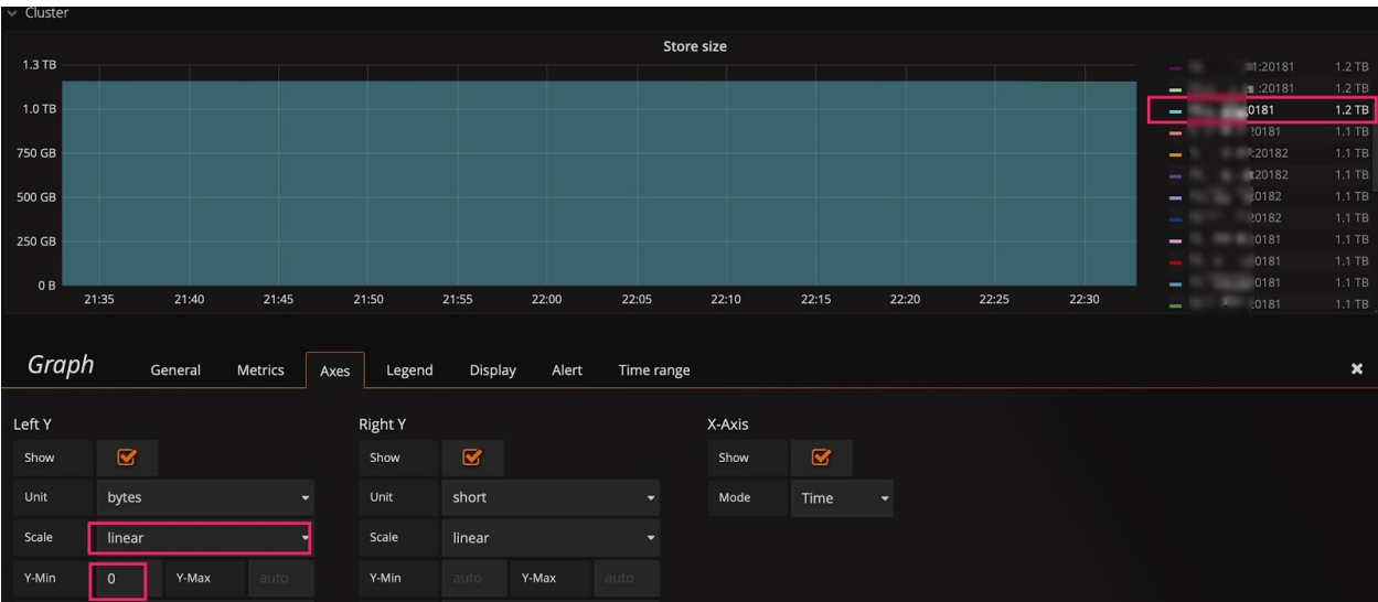
图 29: 基线默认为 0
