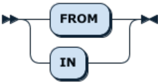
图 126: FromOrIn
