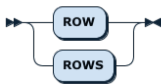
图 94: RowOrRows
