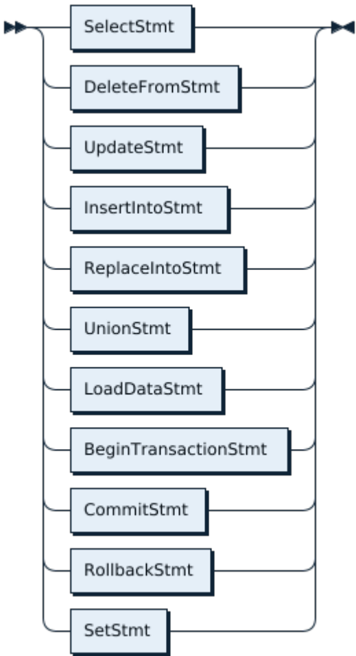
图 198: TraceableStmt
