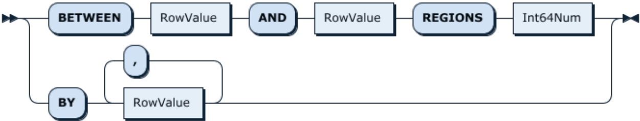
图 194: SplitOption
