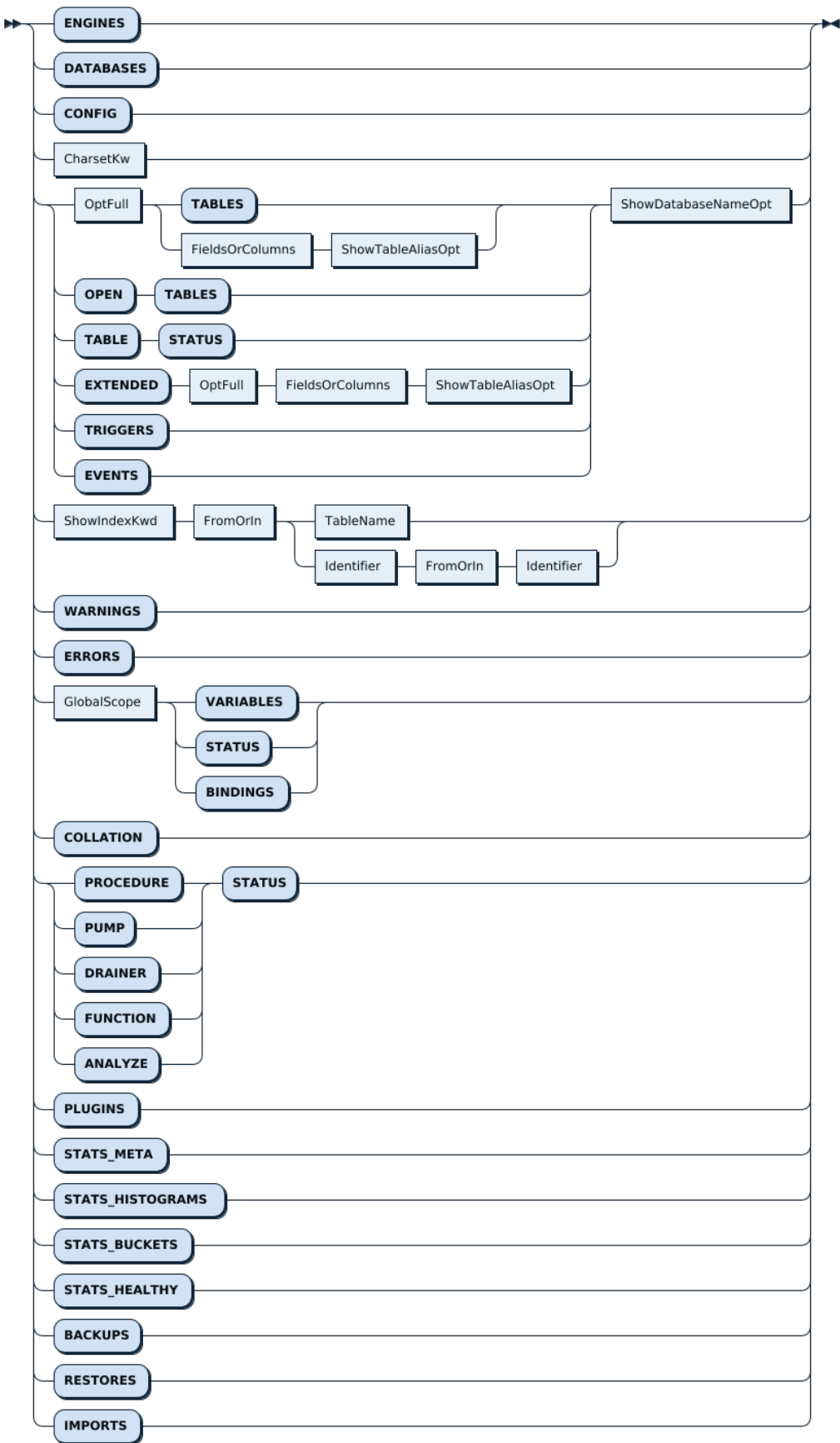
图 132: ShowTargetFilterable
