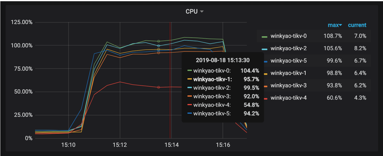
图 19: QPS6
