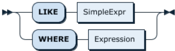
图 184: ShowLikeOrWhereOpt
