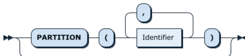
图 175: PartitionNameListOpt
