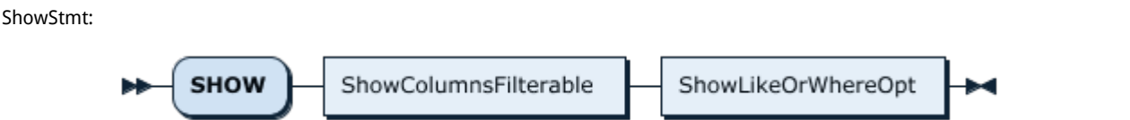
图 155: ShowStmt
