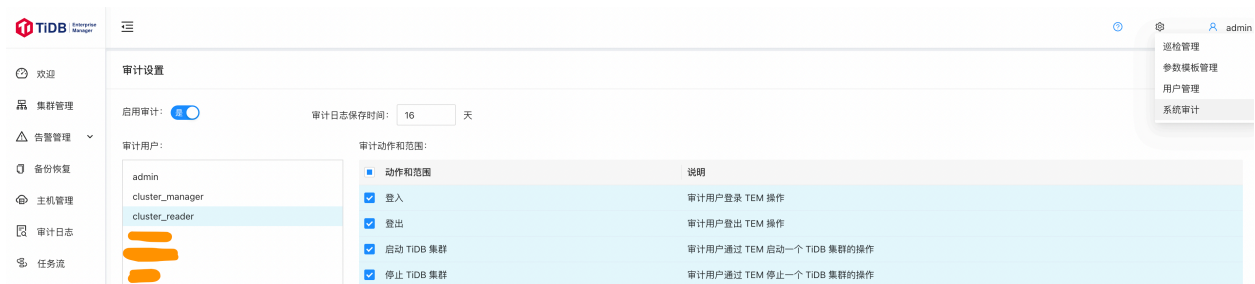
图 255: 审计设置
