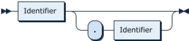
图 127: TableName
