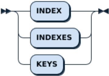
图 149: ShowIndexKwd
