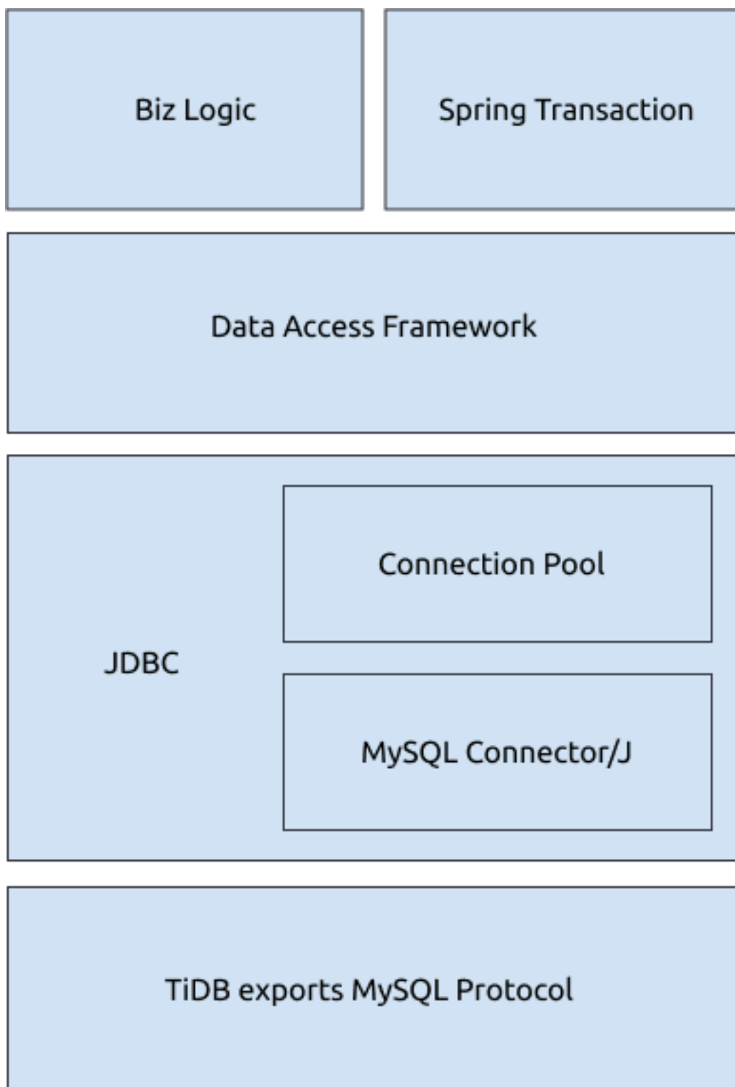
图 9: Java Component
