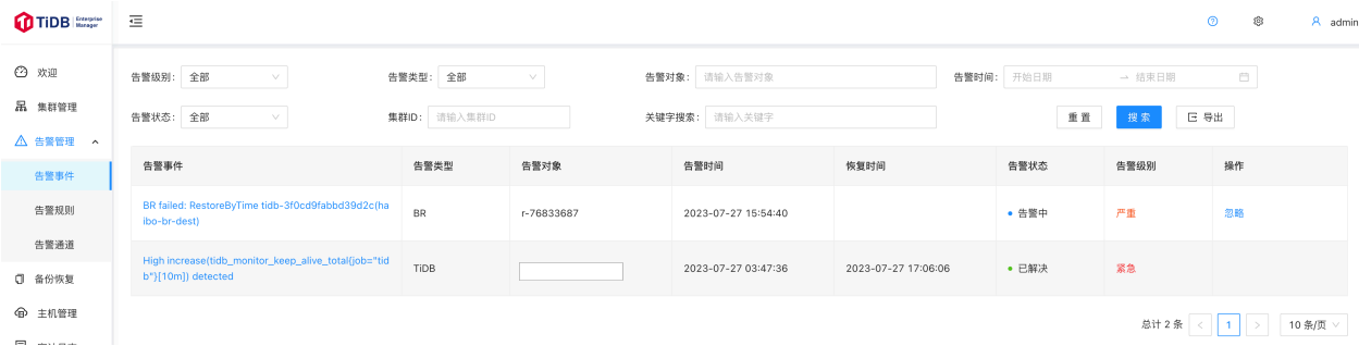
图 246: 告警事件
