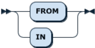
图 179: FromOrIn
