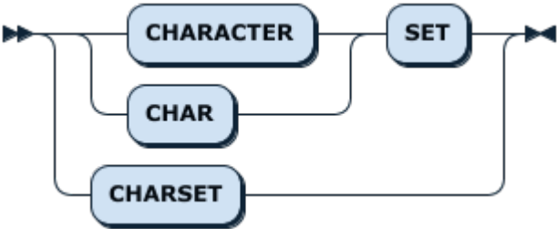
图 105: CharsetKw
