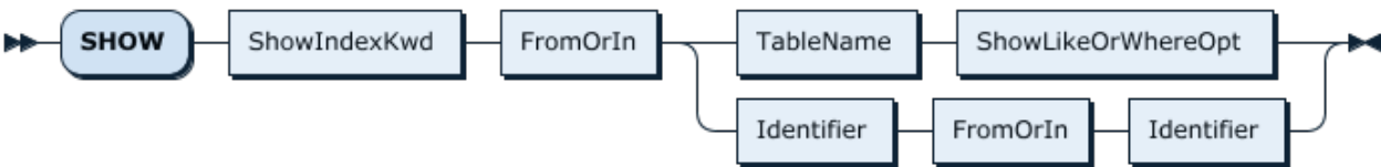
图 148: ShowIndexStmt
