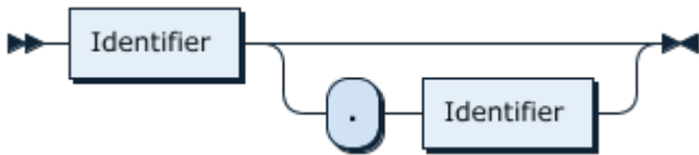
图 134: TableName
