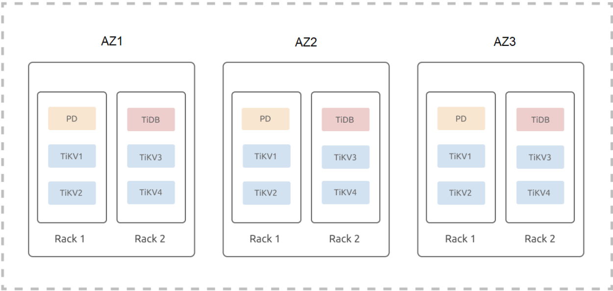
图 4: 同区域三 AZ 集群部署
