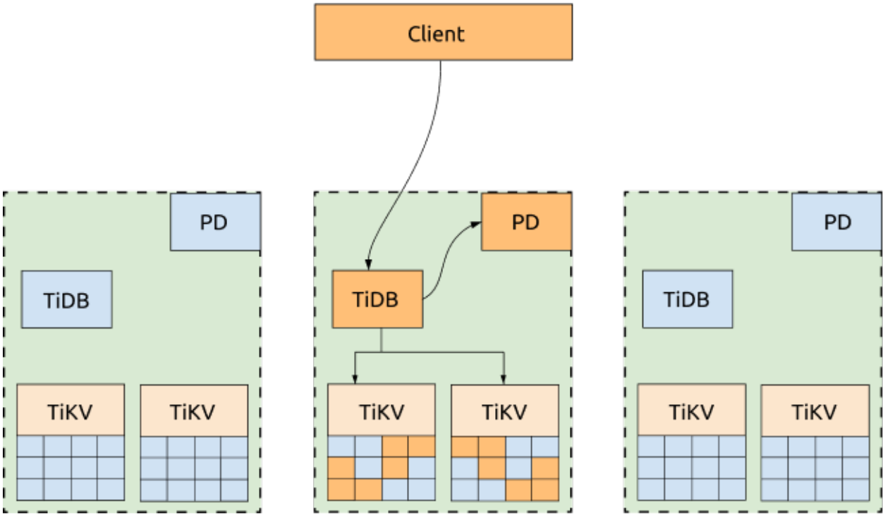
图 3: 三 AZ 部署读性能优化
