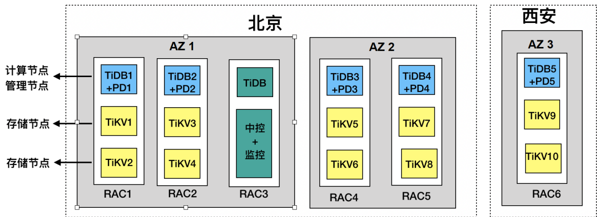
图 6: 双区域三 AZ 配置详图
