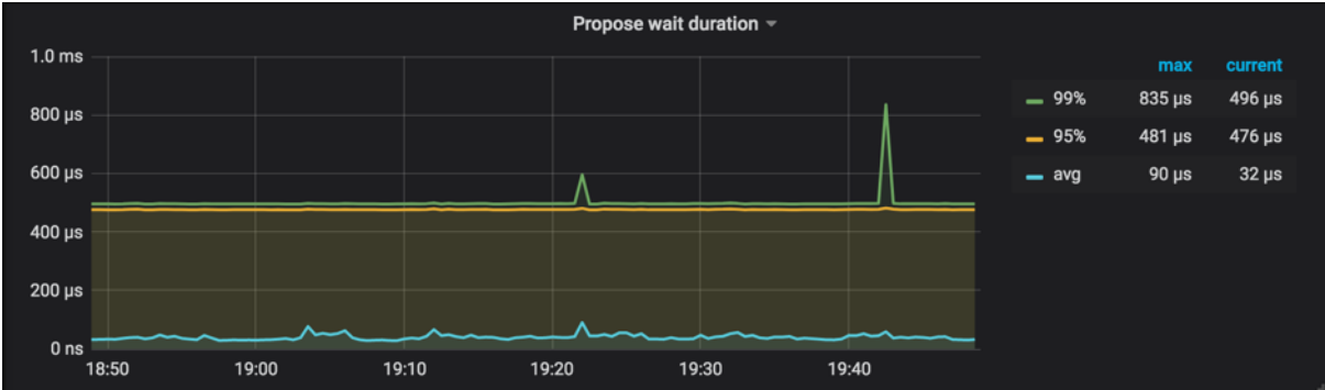
图 40: 图 3 查看 Propose wait duration
