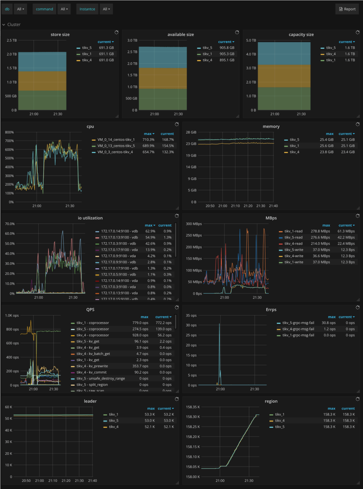
图 64: TiKV Dashboard - Cluster metrics
