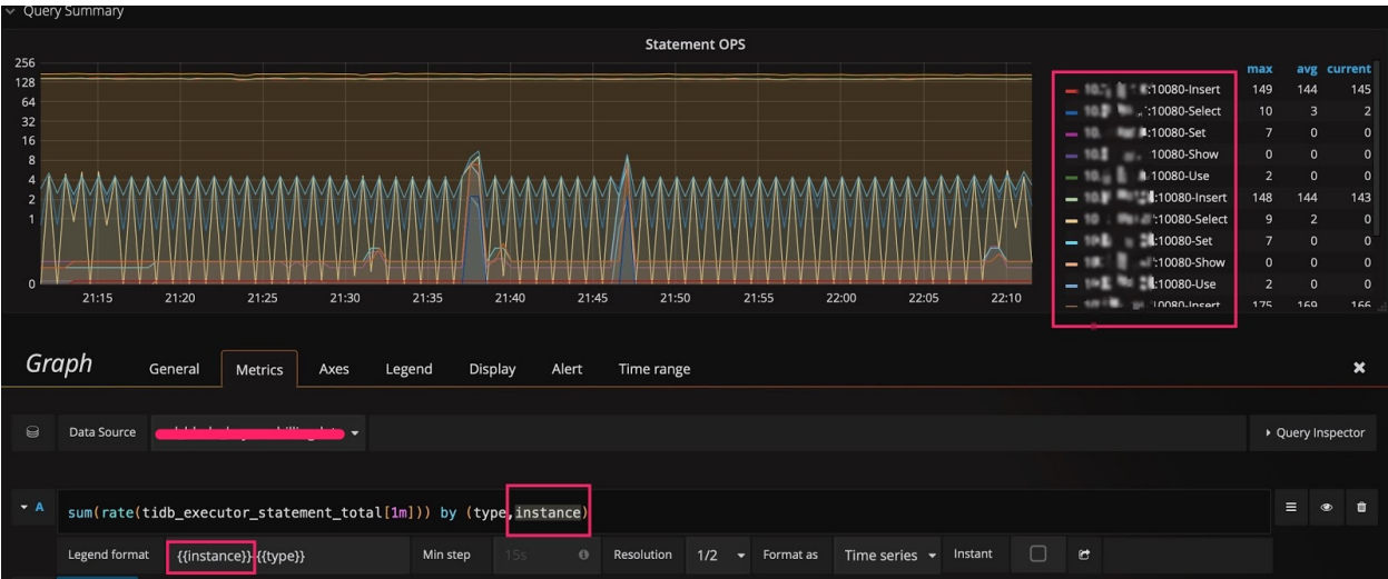
图 26: 给表达式增加一个 instance 维度
