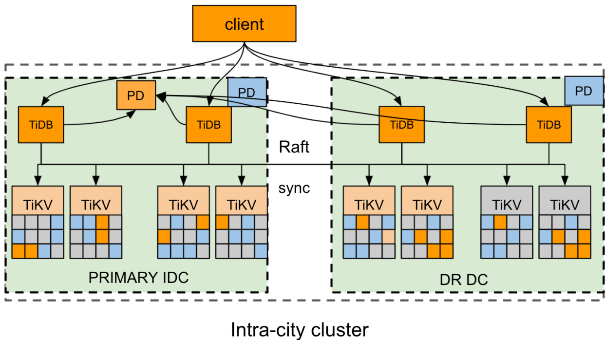
图 8: 单区域双 AZ 集群架构图
