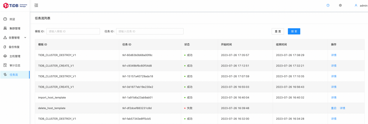
图 257: 任务流管理
