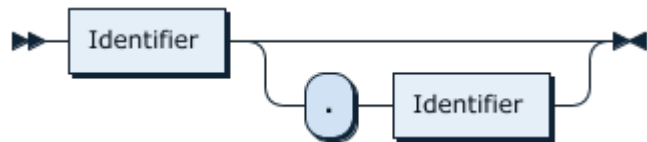
图 172: TableName
