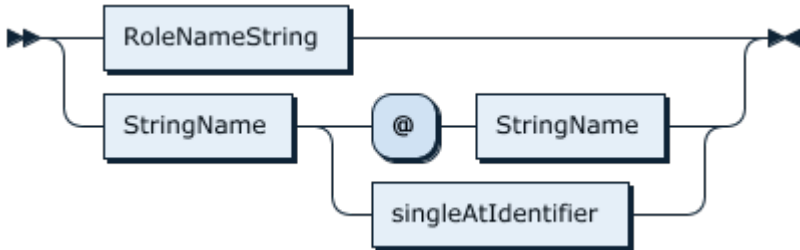
图 147: Rolename
