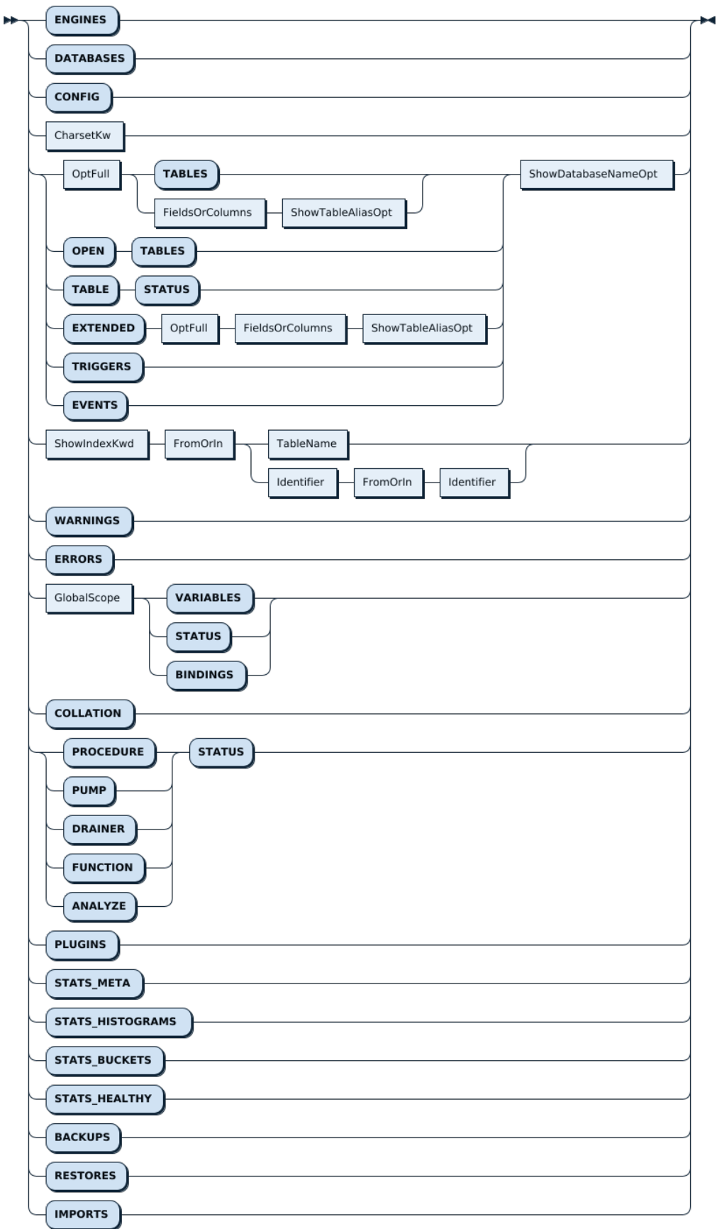
图 160: ShowTargetFilterable
