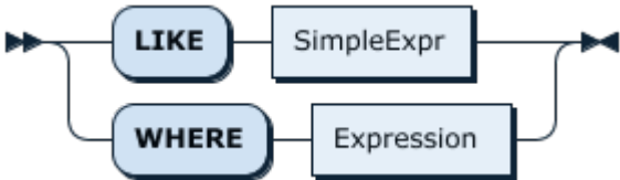
图 130: ShowLikeOrWhereOpt
