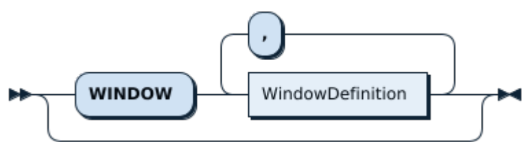
图 95: WindowClauseOptional
