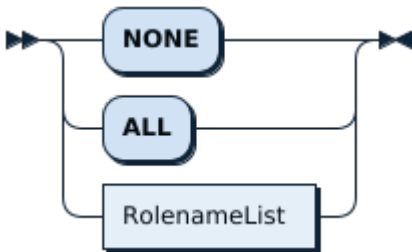
图 97: SetDefaultRoleOpt
