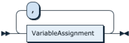
图 101: VariableAssignmentList
