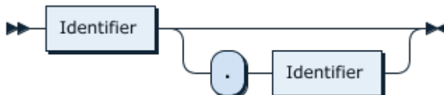
图 136: TableName
