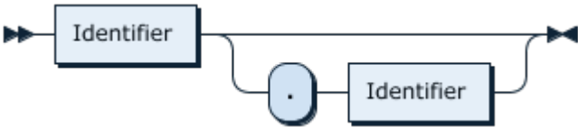
图 192: TableName
