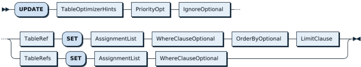
图 204: UpdateStmt
