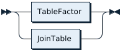
图 206: TableRef
