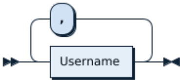
图 99: UsernameList
