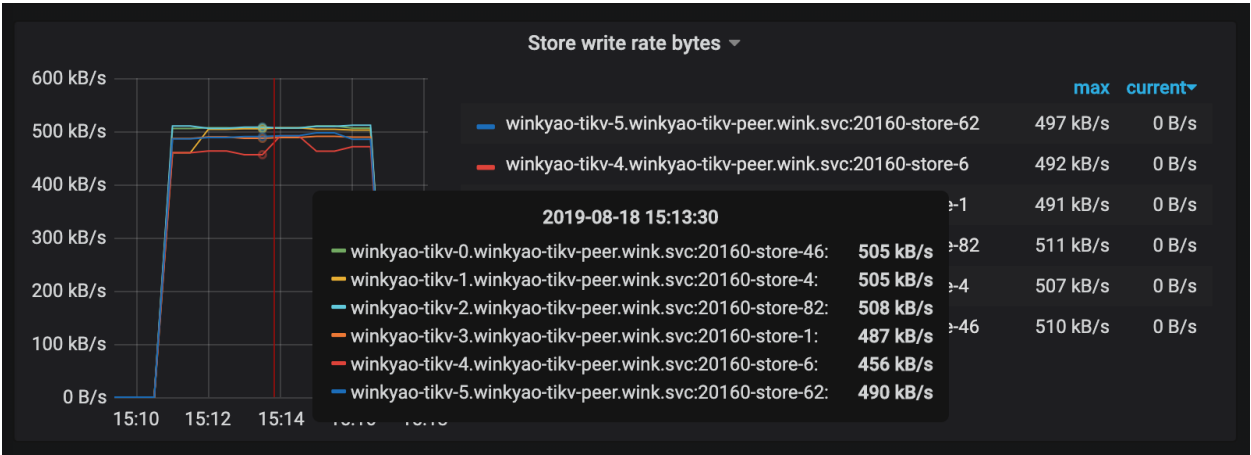
图 21: QPS8
