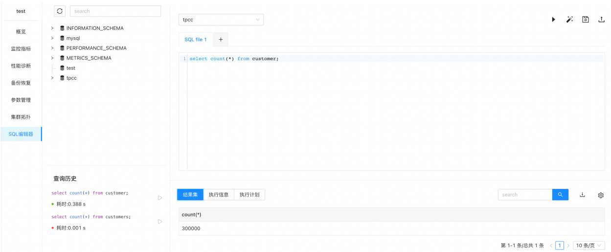
图 236: SQL 编辑器
