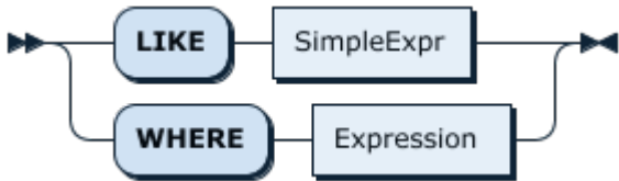
图 140: ShowLikeOrWhereOpt
