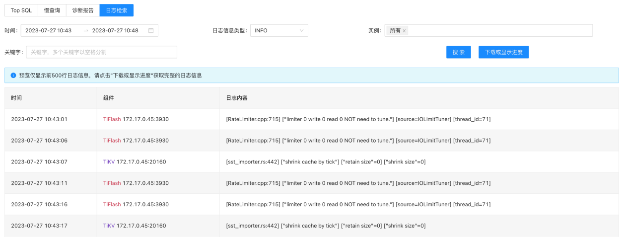
图 231: 日志检索
