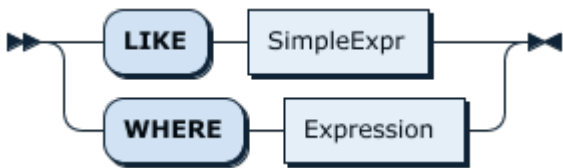
图 161: ShowLikeOrWhereOpt
