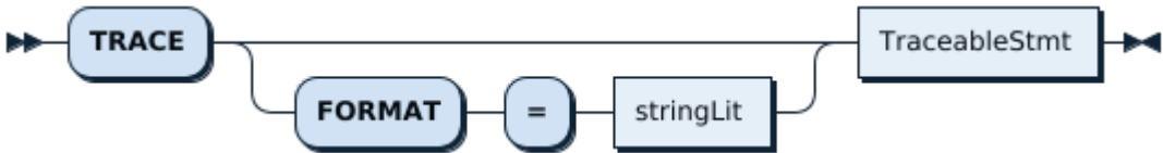
图 197: TraceStmt
