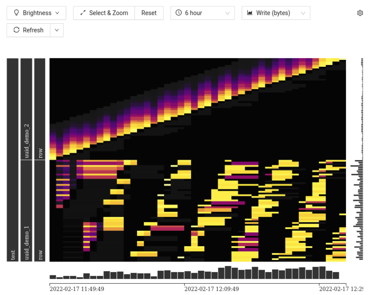
图 47: Key Visualizer
