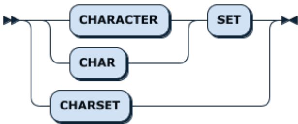
图 119: CharsetKw
