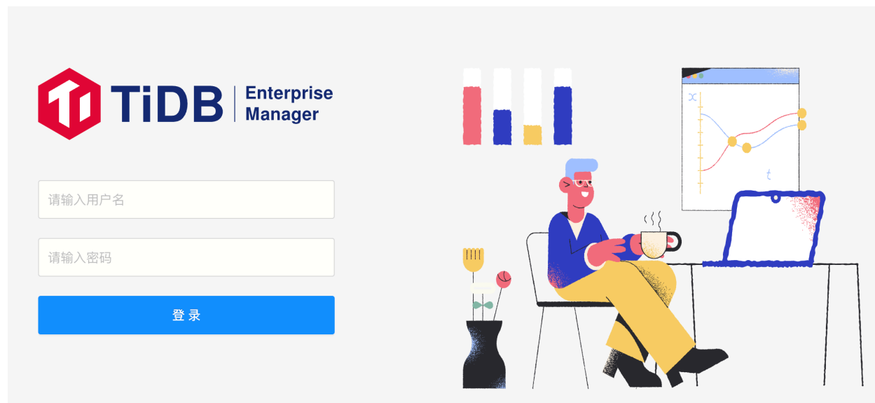
图 218: 登陆页面
