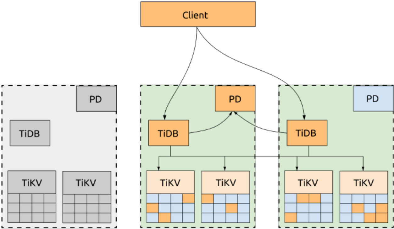
图 2: 三 AZ 部署容灾
