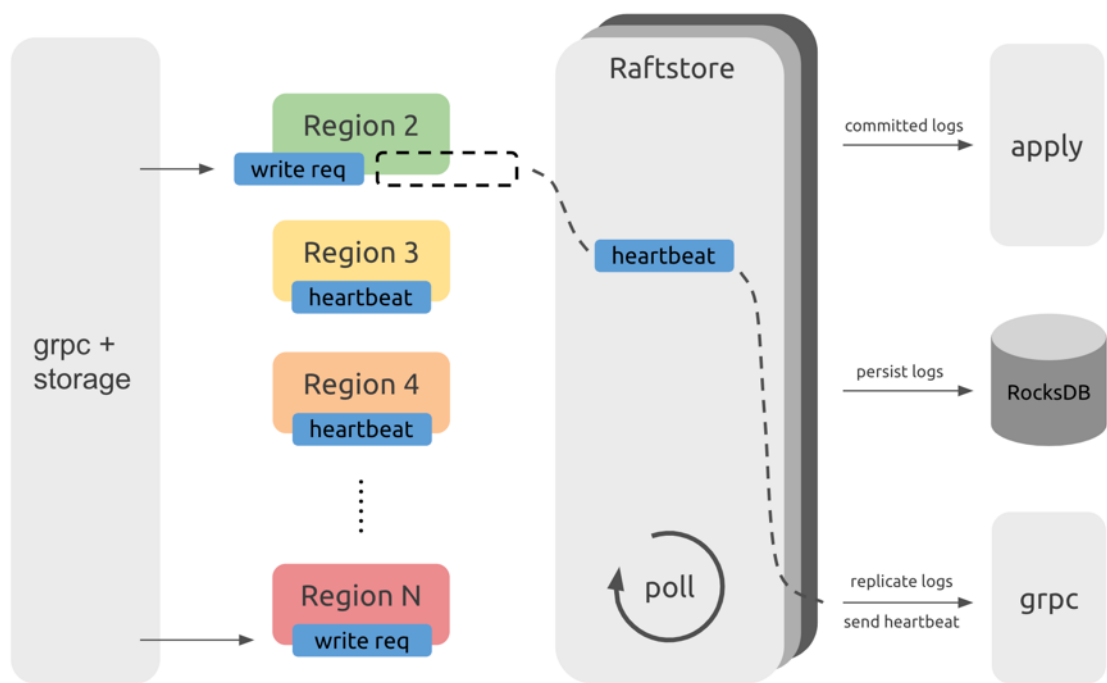
图 38: 图 1 Raftstore 处理流程示意图
