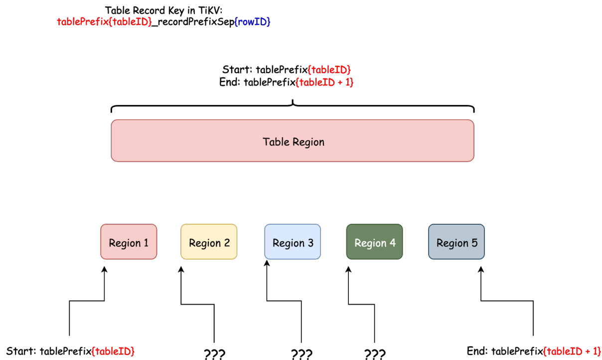
图 18: Table Region Range
