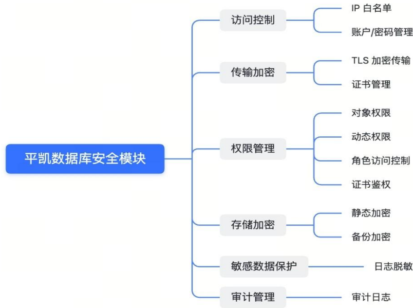
图 2: 平凯数据库 Security
